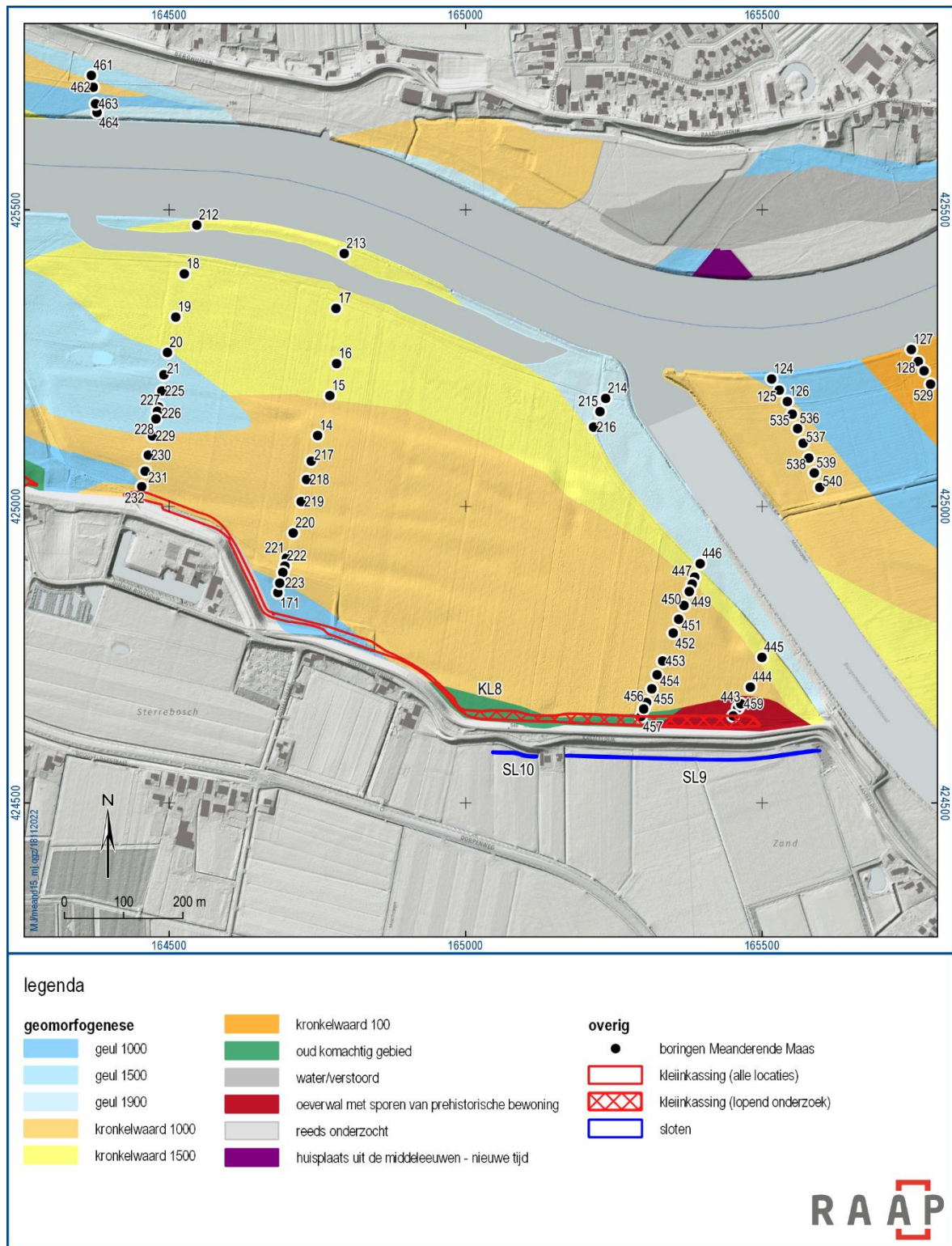
Figuur 8. Geomorfogenese bij Ossekamp (oostelijk deel).
