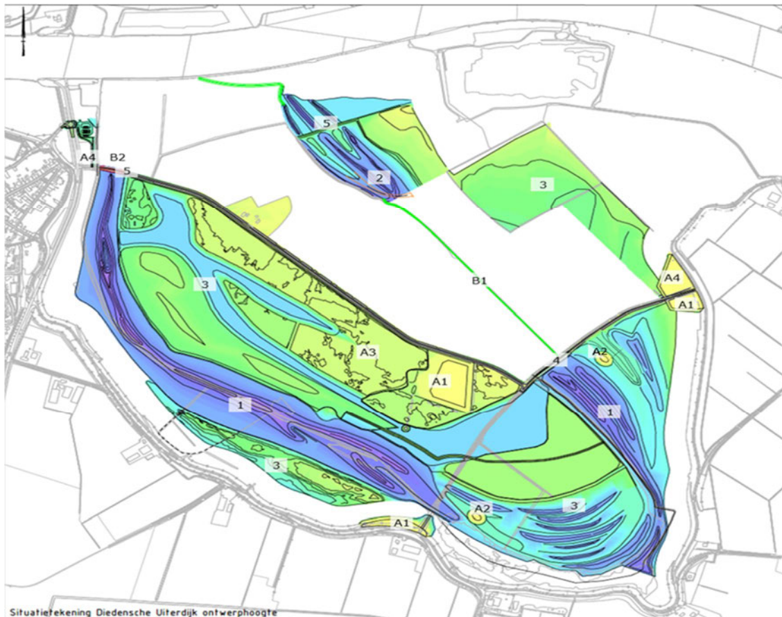
Figuur 4 Ontwerphoogte Diedensche Uiterdijk
