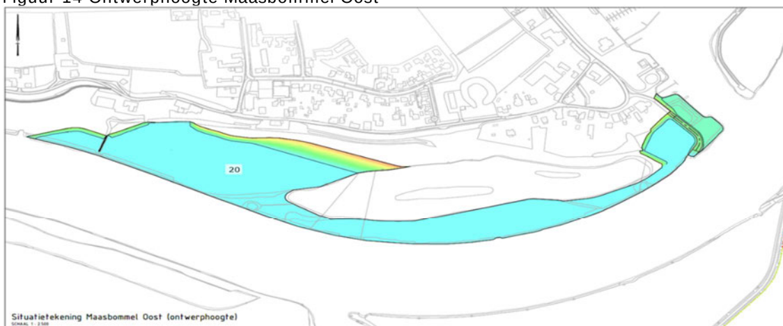
Figuur 14 Ontwerphoogte Maasbommel Oost
