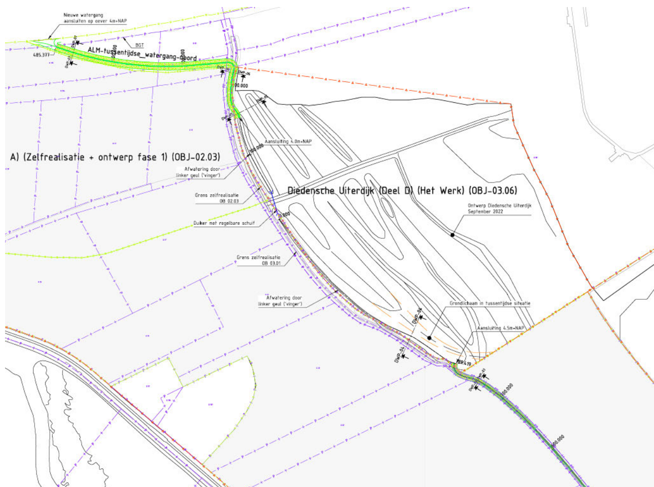
Afbeelding 3.5 Uitsnede van de technische tekening met de uitstroom van de watergang en het raakvlak met de KRW-geulen
