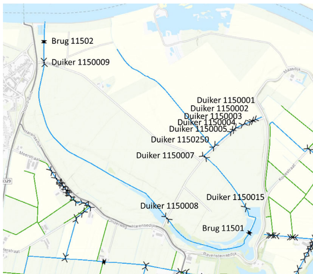
Afbeelding 2.2 Ligging van duikers en bruggen in de Diedensche Uiterdijk - huidige situatie
