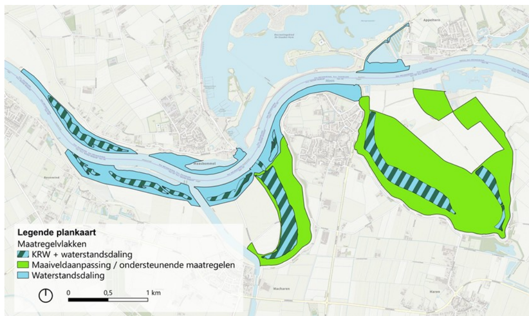
Afbeelding 3.1 Ruimtebeslag van Projectplan Waterwet Rivierverruiming en KRW Meanderende Maas van Rijkswaterstaat
