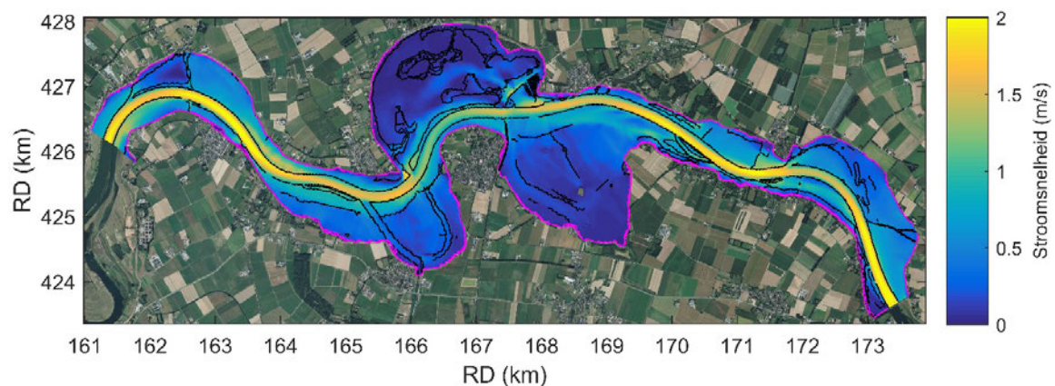
Afbeelding 4.2 Absolute stroomsnelheid (m/s) van het ontwerp in 2D bij een afvoer van 4.118 m 3 /s te Borgharen
